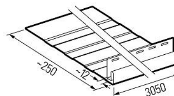
SV(P) 19 Destello de fachada largo
