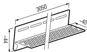
SV(P) 14 Perfil final
