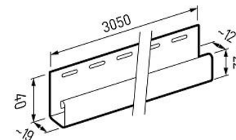
SV(P) 15 Perfil J
