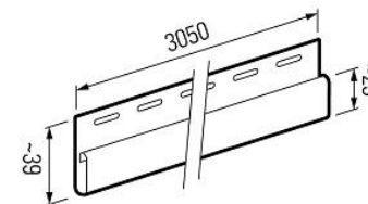
SV(P) 14 Perfil final
