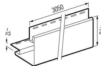
SV(P) 15 Perfil J
