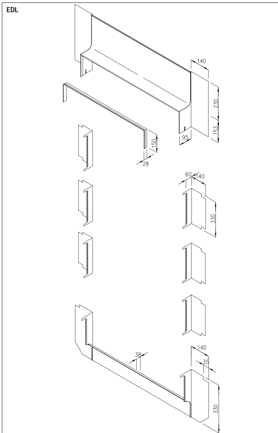
Cercos para materiales de cubierta planos
