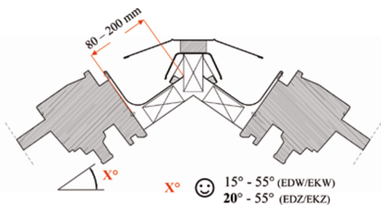
Detalle de encuentro en cumbre
