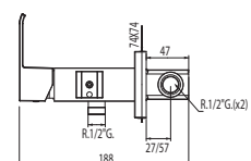
Monomando empotrar para bidé WC Ducha de latón con racord limitador 5 l/m. Antigoteo y flexo SATIN
